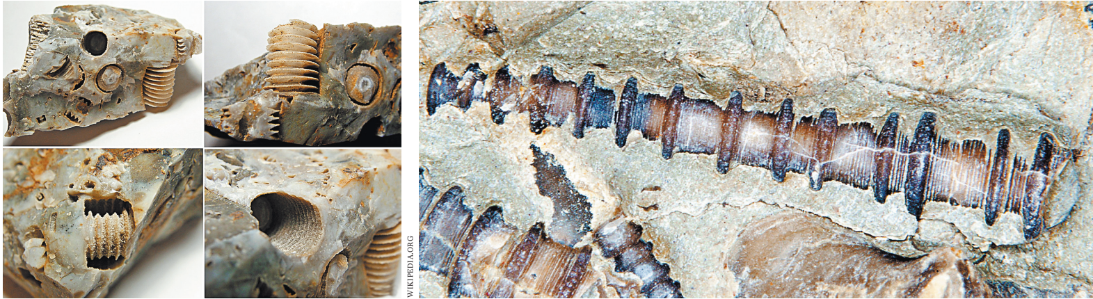
Фото № 2: когда вам будут показывать такие «винты» и «шурупы», знайте, что это криноидеи (слева) и тентакулиты.
